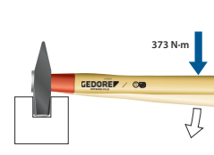
Biegefestigkeit
