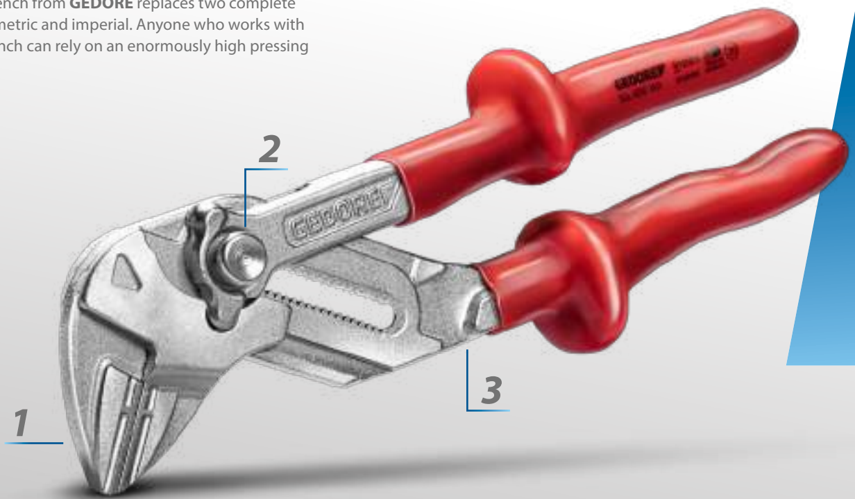
VDE Pliers wrench VDE 183 10
